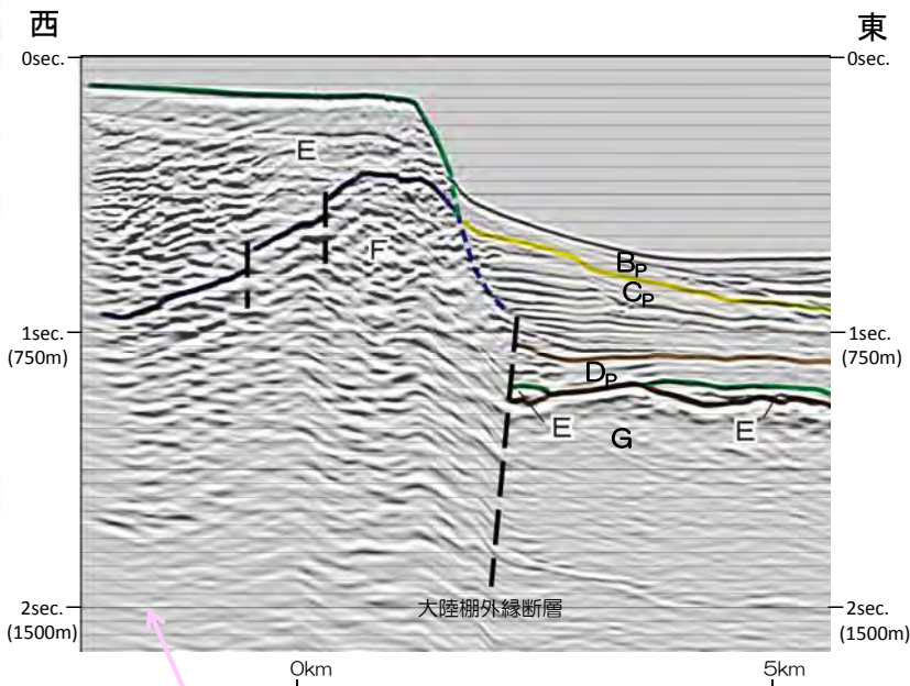
【12ML-O1測線】
