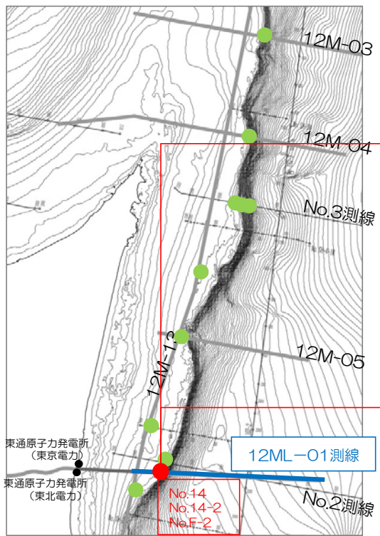
採泥調査位置図
