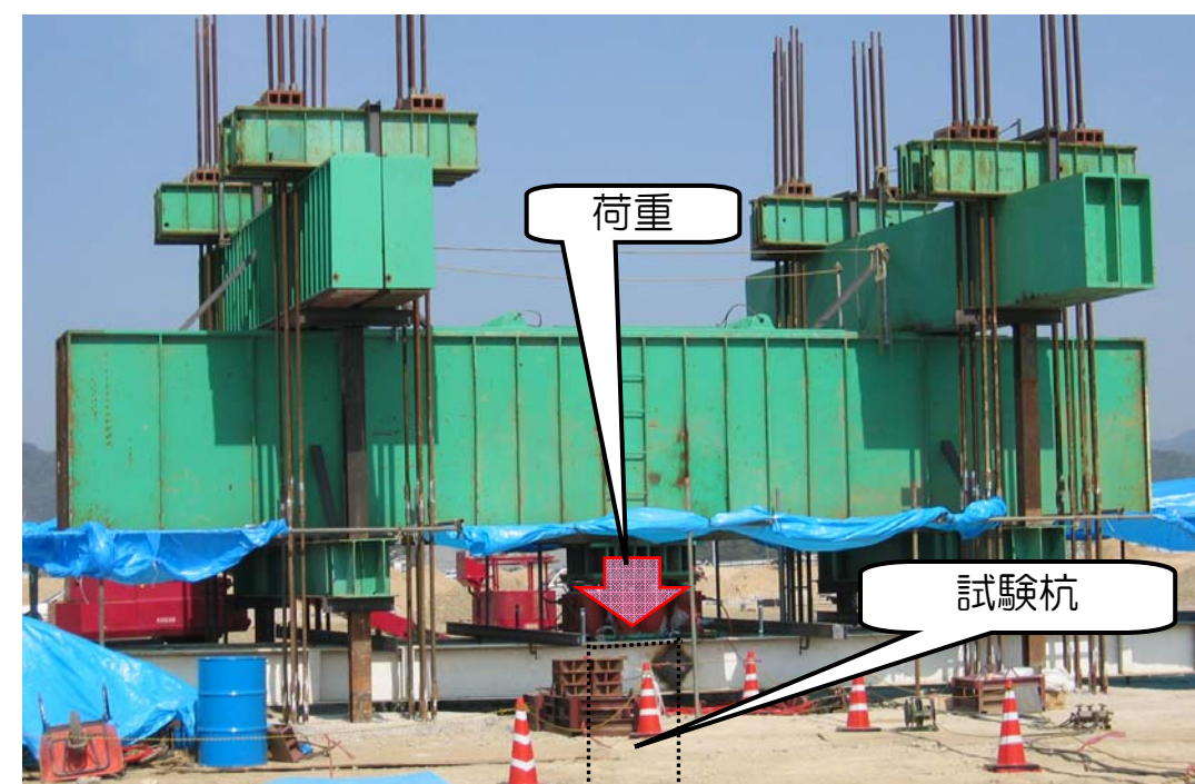
杭の載荷試験(イメージ)
