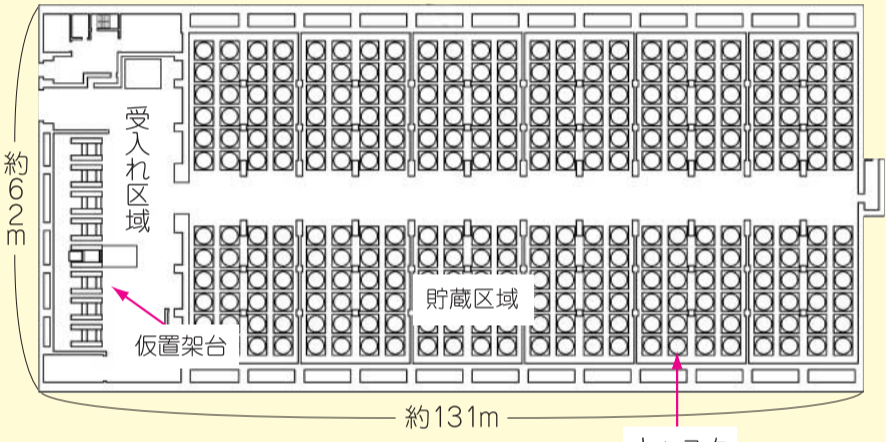
【貯蔵建屋平面図】
