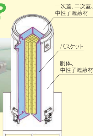
金属キャスクイメージ図
