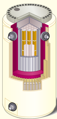
金属キャスクイメージ図
